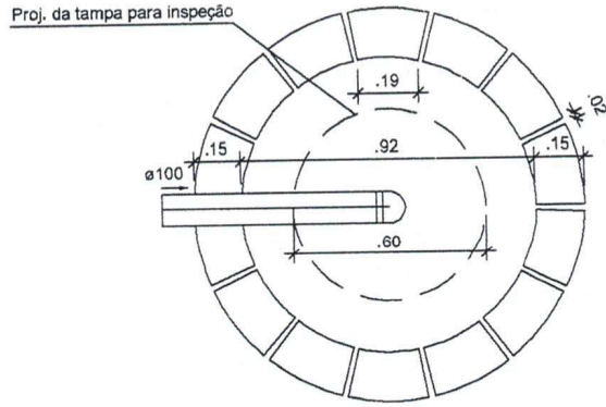
SUMIDOURO - PLANTA-BAIXA ESCALA 1/ 25
