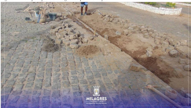
Figura 3 - Recuperação e drenagem de pavimentação
