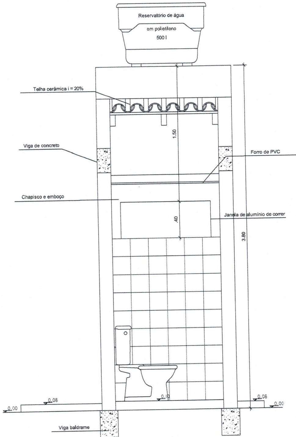
○ CORTE BB ESCALA 1/25
